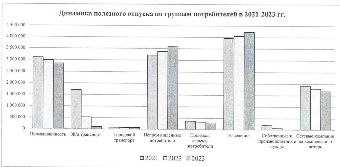
Рисунок 1 - Динамика полезного отпуска 2021-2023 гг. по группам потребителей, тыс. кВтч
